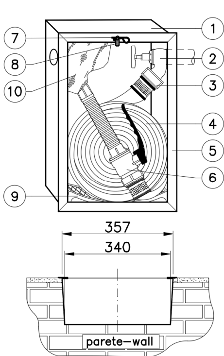
Vista inferiore – Bottom view
